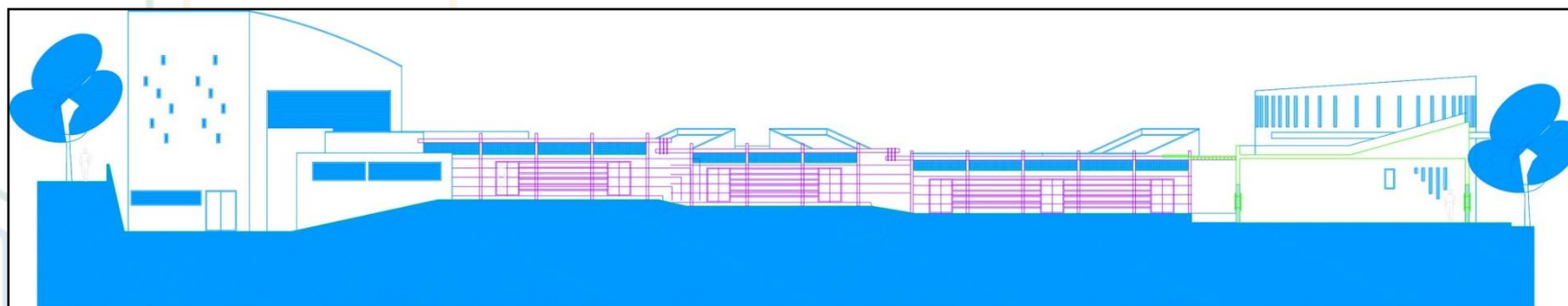
ELEVACIÓN NORTE ESCALA 1:100
